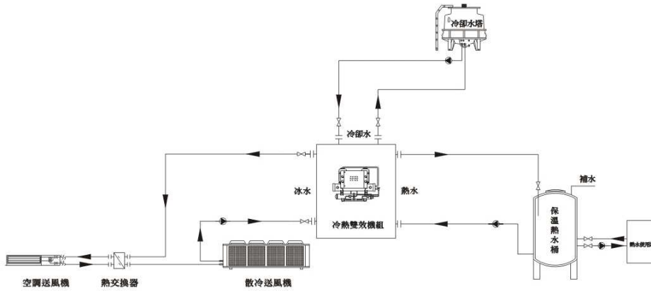
■ 冷熱雙效系統流程圖
